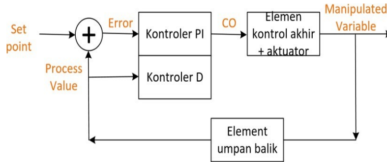
Gambar 8. Kontroler PID yang disempurnakan
