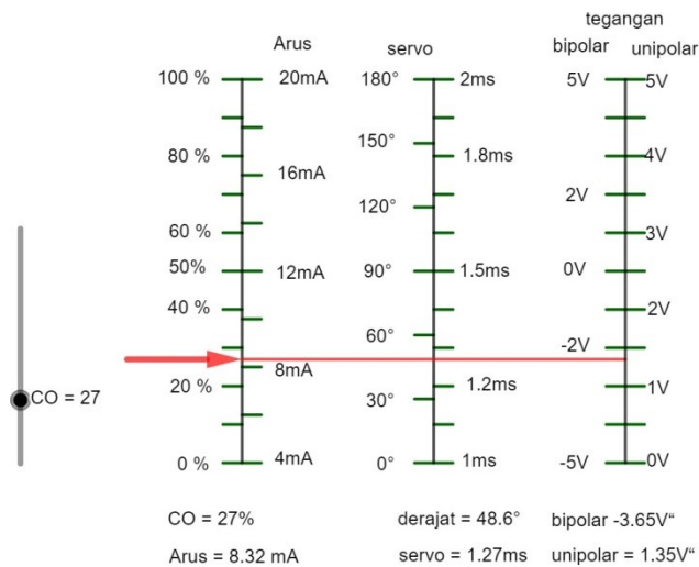
Gambar 4. Pemetaan untuk CO menjadi keluaran yang diinginkan
