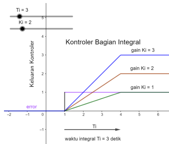
Gambar 6. Pengaruh Kontroler bagian integral
