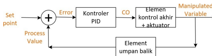
Gambar 2. Diagram blok Pengendali PID
