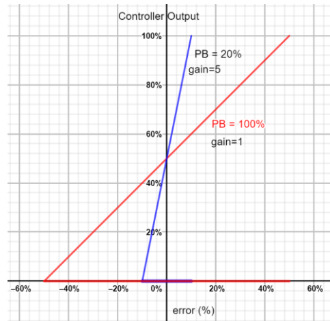
Gambar 5. Proporsional Band, error dan Keluaran Kontroler
