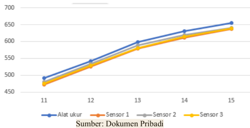
Gambar 22. Grafik hasil sensor menyebarkan CO 2 di bagian tengah box
