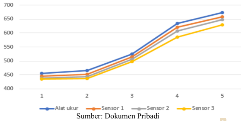
Gambar 20. Grafik hasil sensor menyebarkan CO 2 di bagian kiri box
