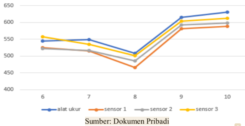
Gambar 21. Grafik hasil sensor menyebarkan CO 2 di bagian kanan box
