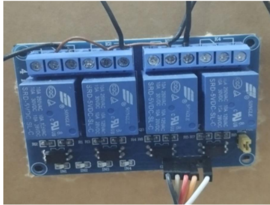
Gambar 15. Pengujian Relay Dengan Tegangan Listrik Mati
