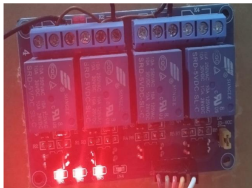
Gambar 16. Pengujian Relay Dengan Tegangan Listrik Hidup
