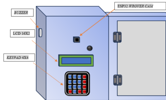
Gambar 3.3 Desain 3D alat
