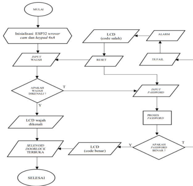
Gambar 3.2 Flowchart kerja alat
