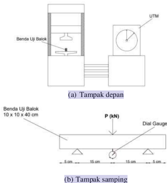
Gambar 1. Set Up Pengujian Keuletan
