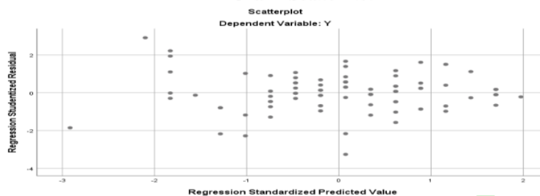
Gambar 2 Grafik ScatterPlot
