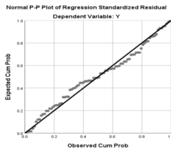
Gambar 1 Grafik P-Plot
