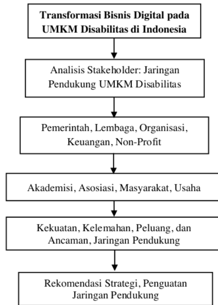
Gambar 1. Kerangka penelitian
