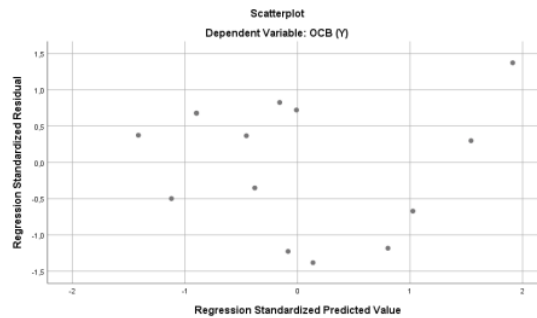
Gambar 1. Grafik Scatterplot
