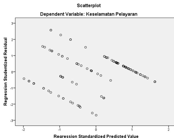
Gambar 2 Grafik Uji Scatterplot
