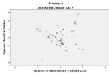
Gambar 1 Uji Heteroskedastisitas
